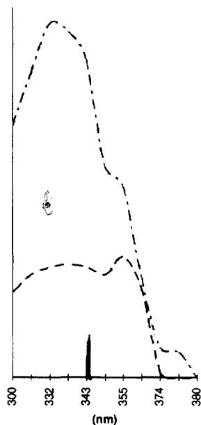
Figure 8. UV absorption: \text{Ca}^{2+} (100 \mu\text{M} ) (—); compound 5p (100 \mu\text{M} ) (---); \text{Ca}^{2+} + 5p (- · - · -).
